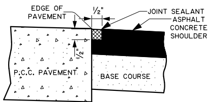
SECTION I-I TYPE PJ (HOT POURED SEALANT SECTION 1005)
