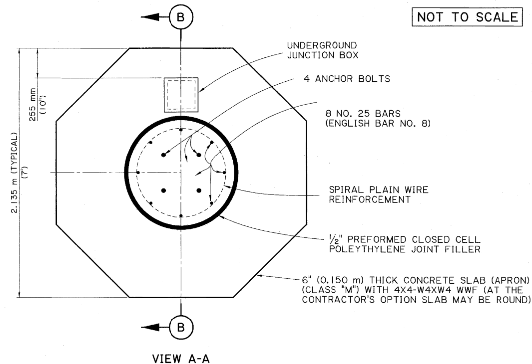
VIEW A-A
