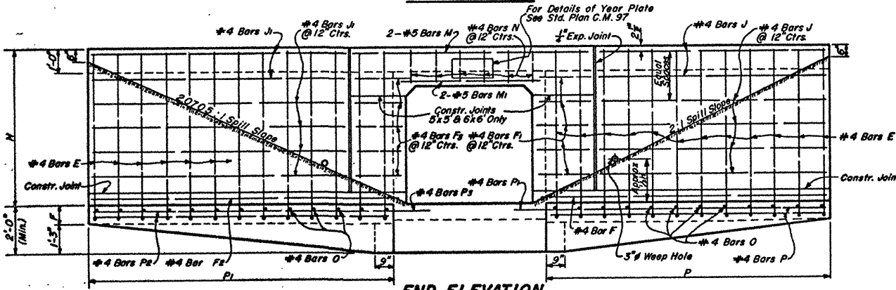
END ELEVATION
