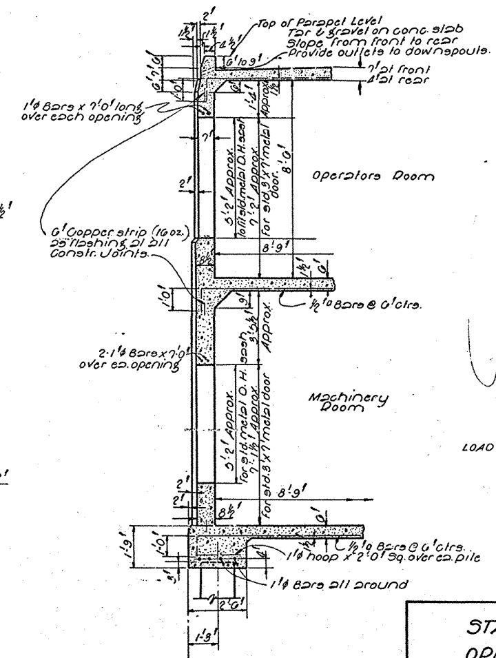
SECTION A-A
