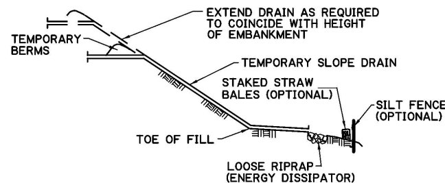
ELEVATION
